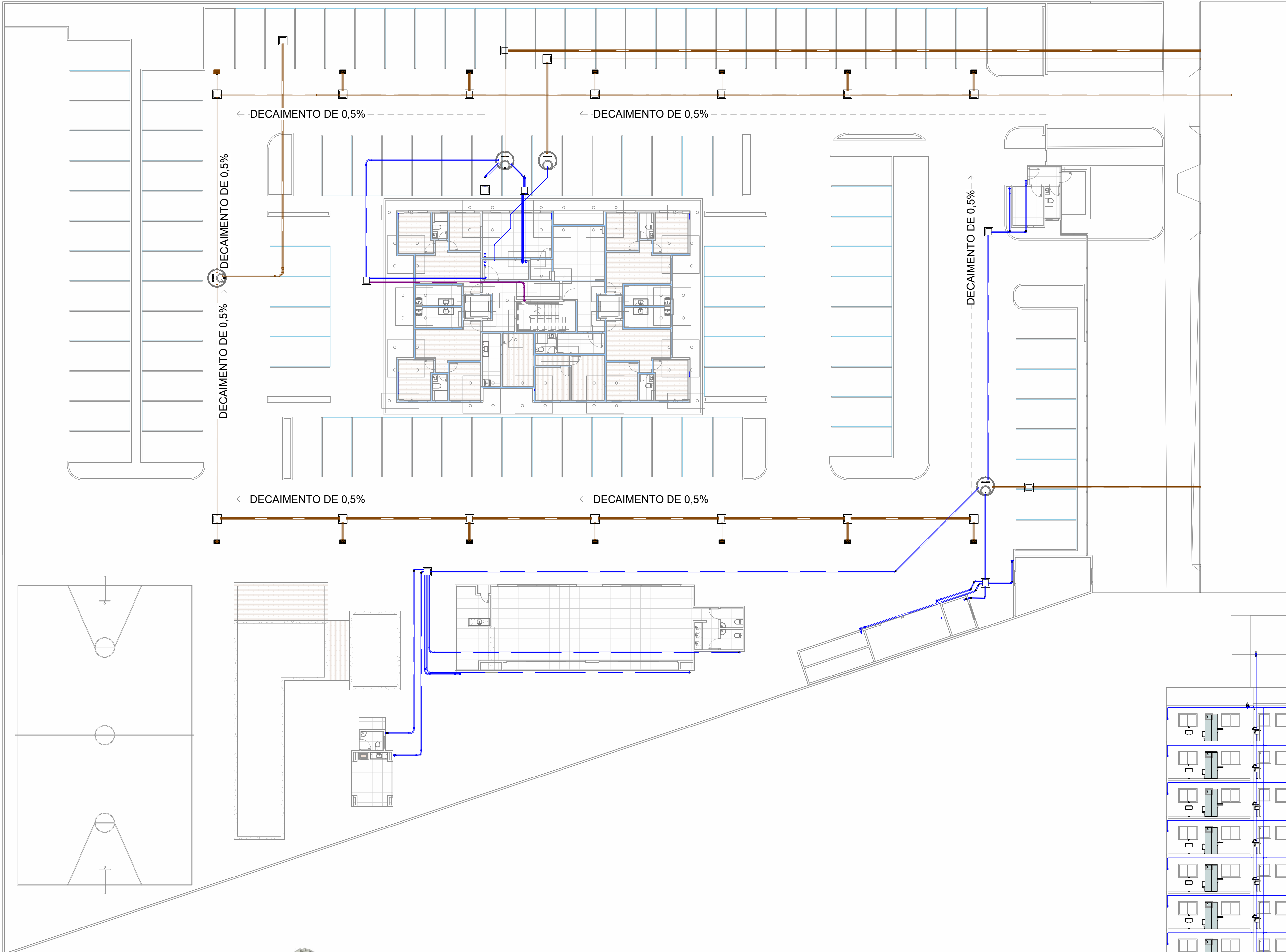
Plano Geral 1 : 200
