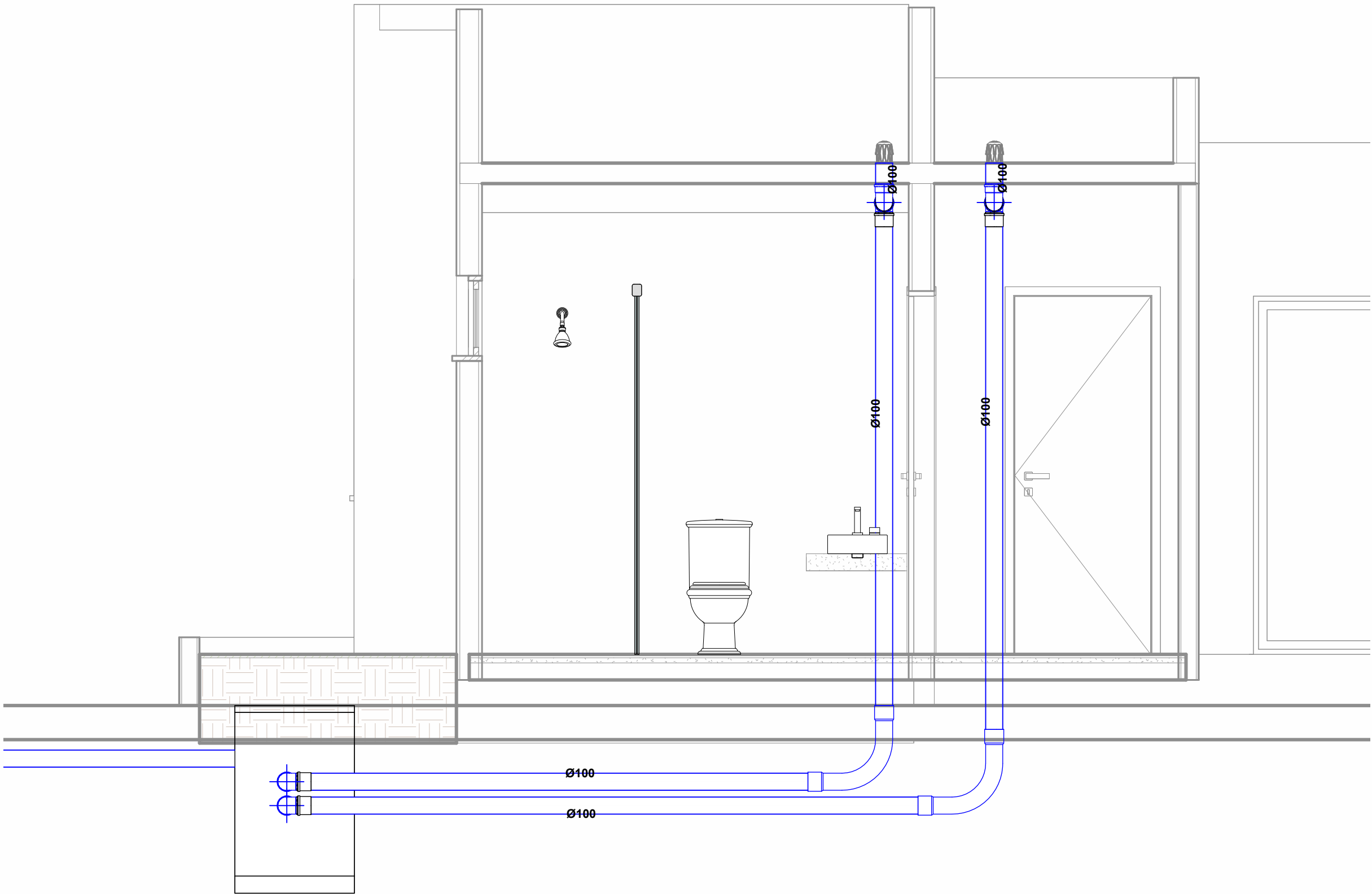
Elevação Guarita 1 : 25
